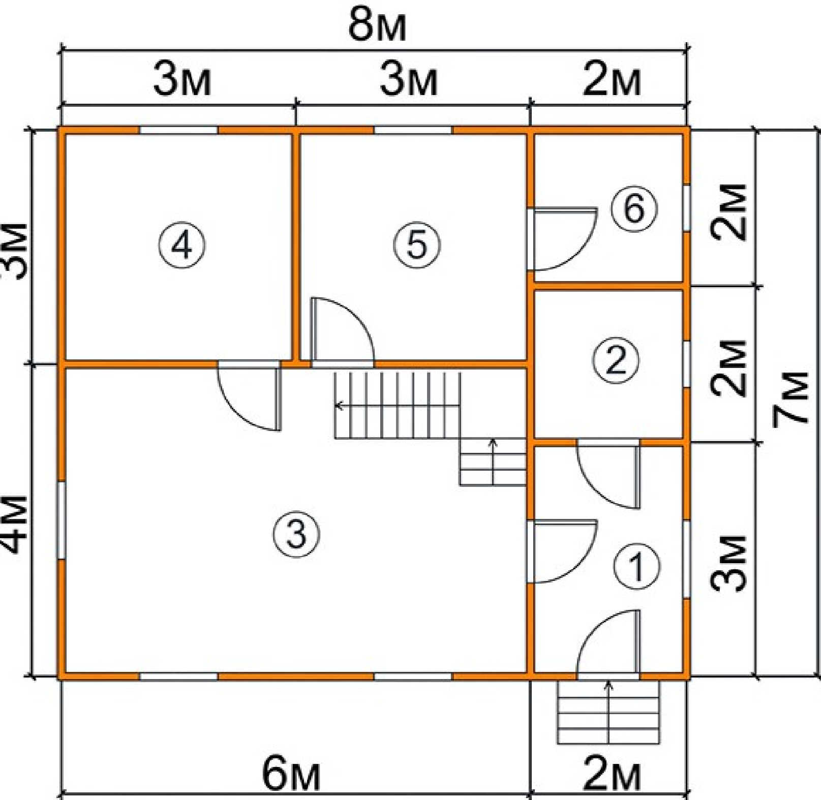
Экспликация помещений
